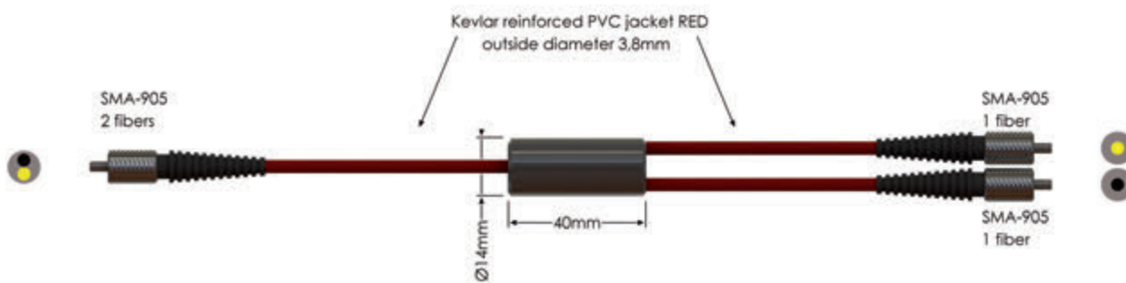
FCB-UVIR400-2
